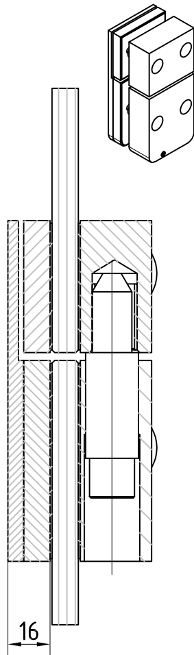
TA nach ausßen öffnend Art. Nr. 04.208
