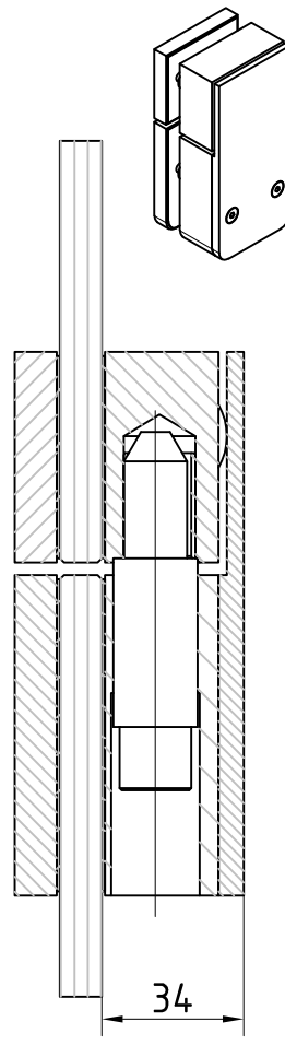
TA nach innen öffnend Art. Nr. 04.209
